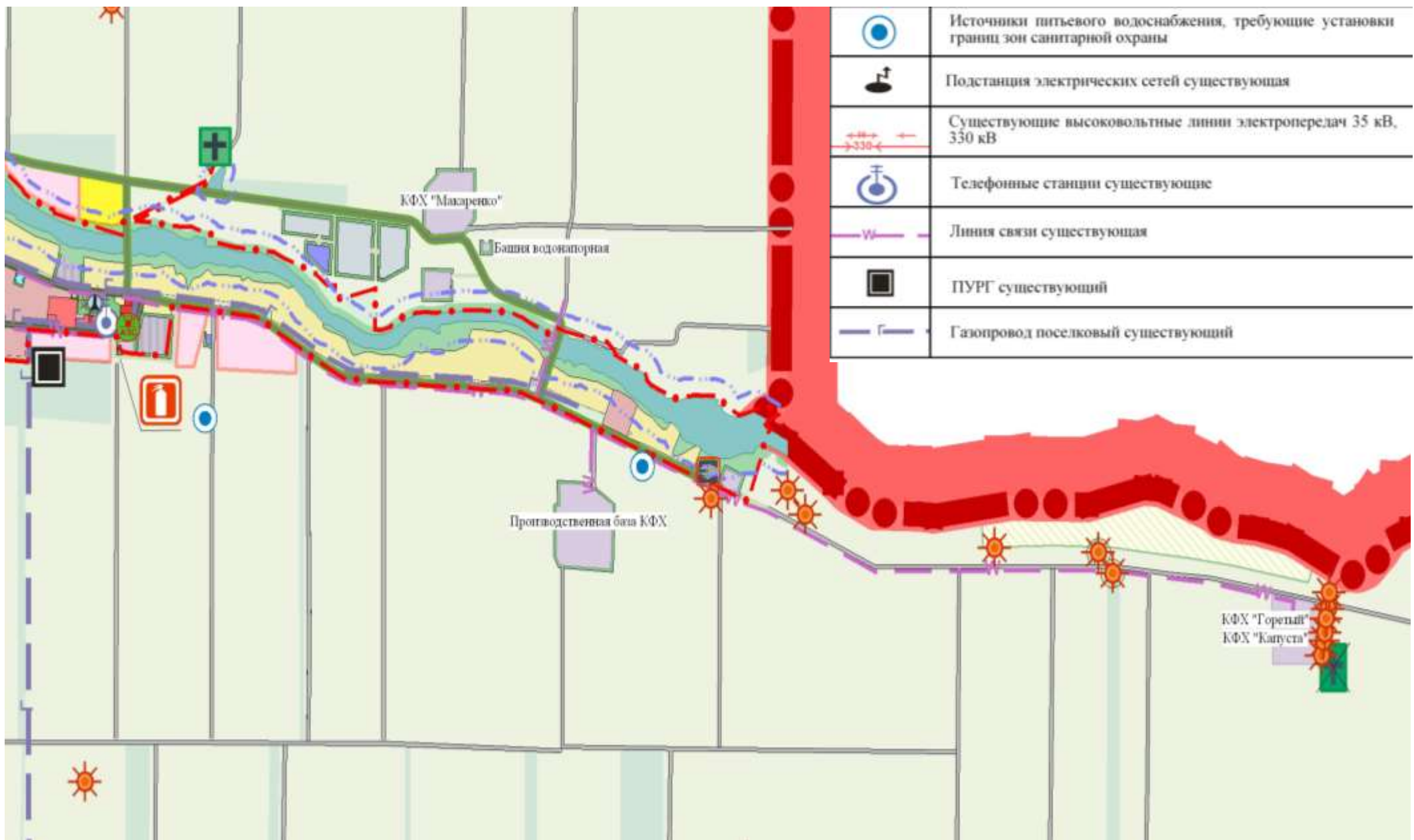
Основной план инженерной инфраструктуры. Существующее состояние.
