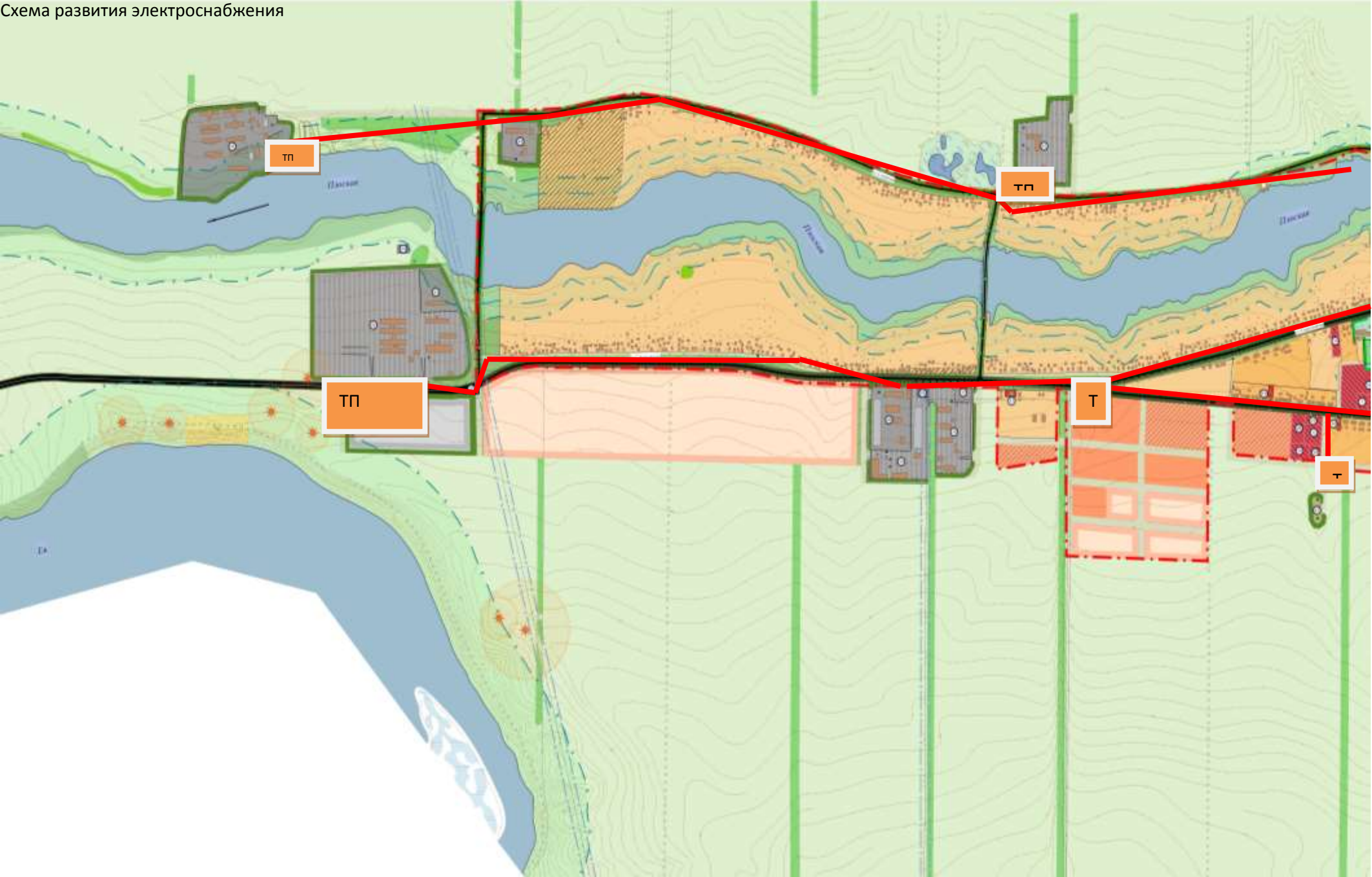
Схема развития электроснабжения
